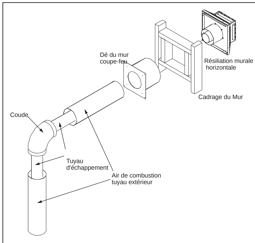
Figure 52: Terminaison d'évent horizontal
