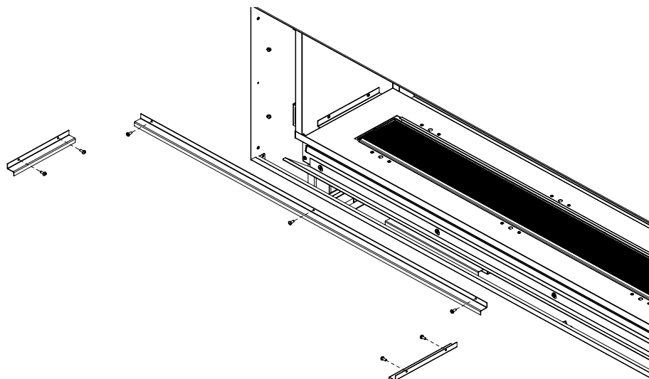
Figure 66: L'installation du panneau
