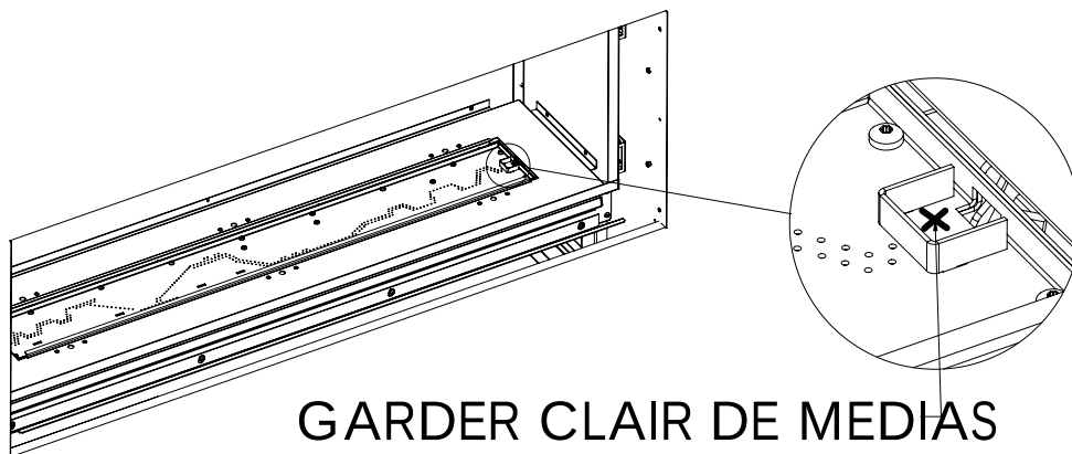
Figure 65: Zone du veileuse protégée
