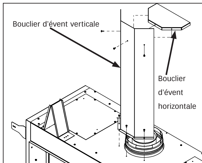
Figure 38: Instalation du bouclier d'évent
