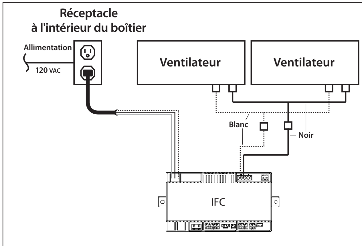
Figure 61: Schéma de câblage du kit d'éclairage. Voir le manuel d'instructions 50-3211 pour le schéma de câblage C44ID
