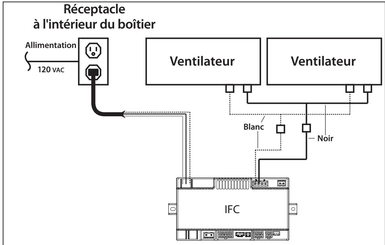
Figure 60: Schéma de câblage du kit de ventilateur C44I. Voir le manuel d'instructions 50-4173 pour le schéma de câblage C44ID
