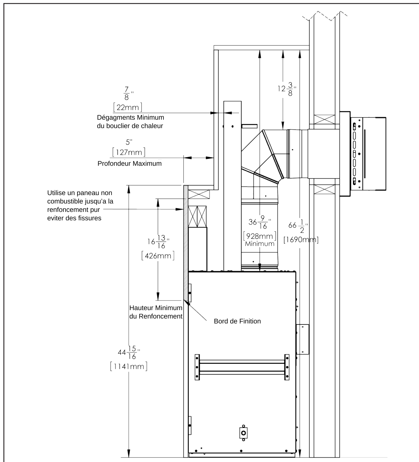
Figure 36: Dimension d'Installation du Renforcement
