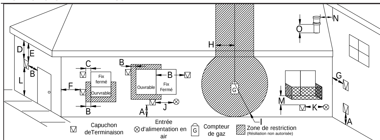
Figure 46: Résiliation d'évent des restrictions, reportez-vous à Tableau 3
