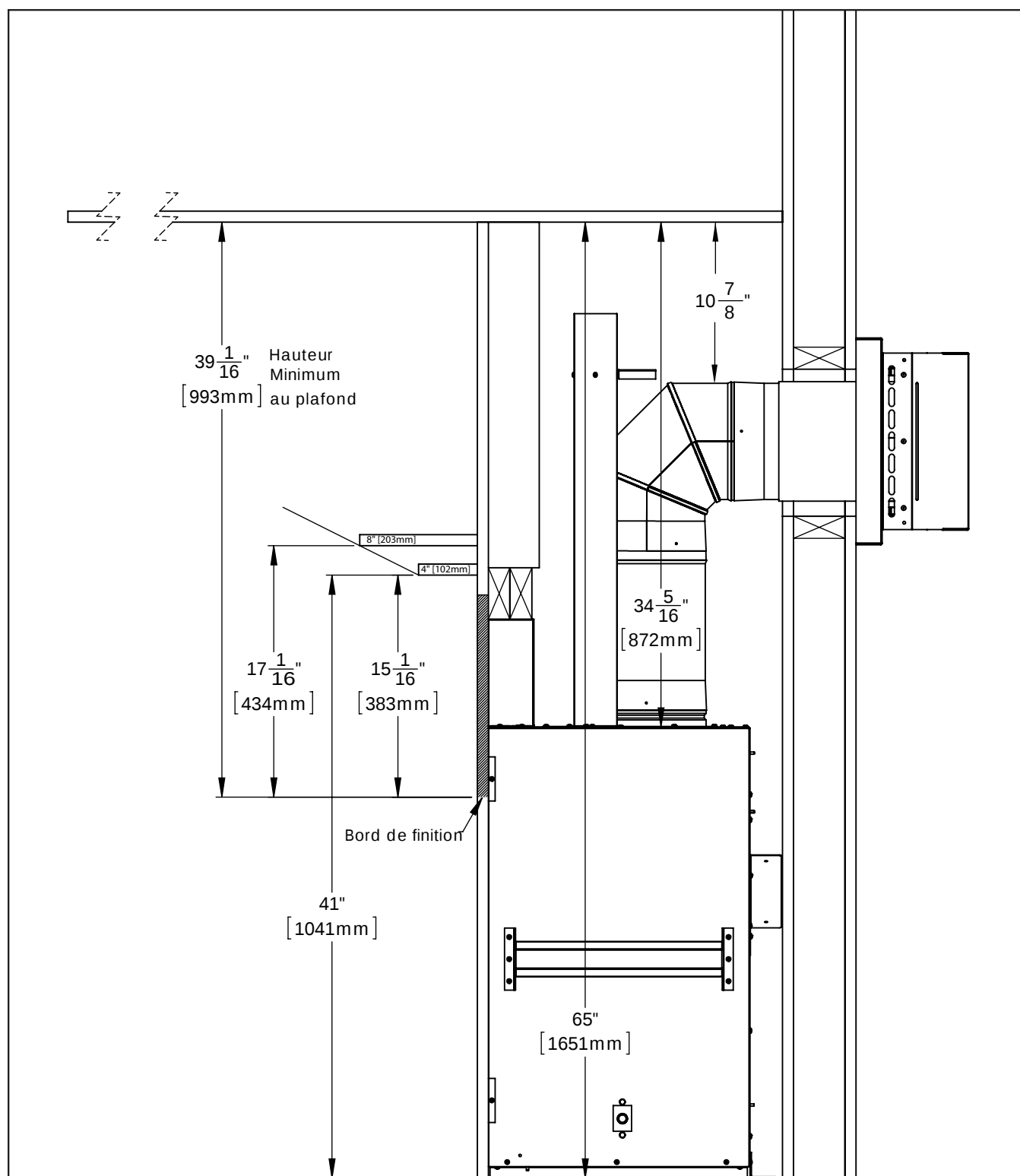
Figure 35: Dimension d'Installation avec Menteau
