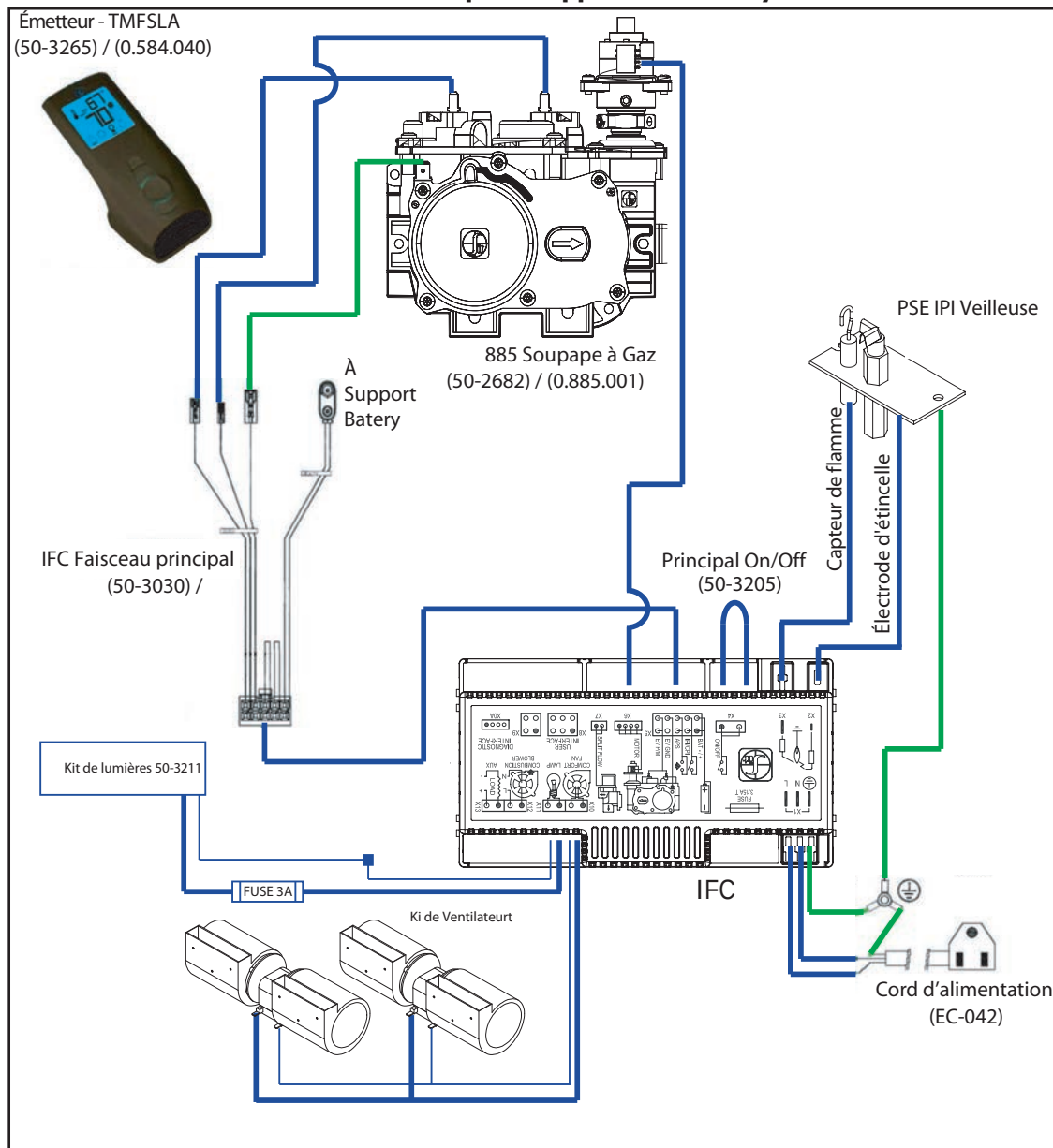
Figure 58: C44I Schéma de câblage
