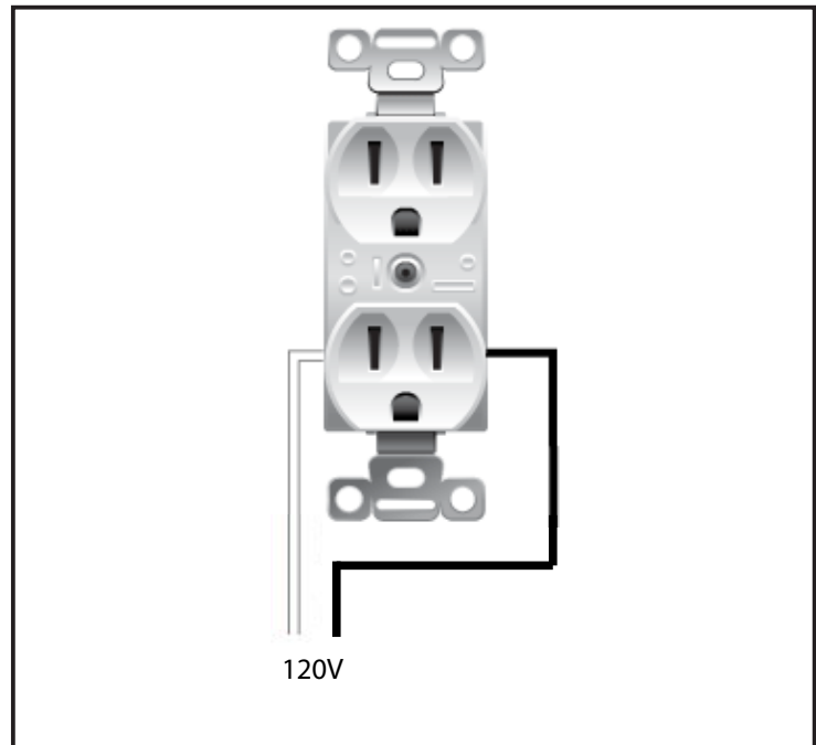
Figure 59: C44I Câblage de la prise
