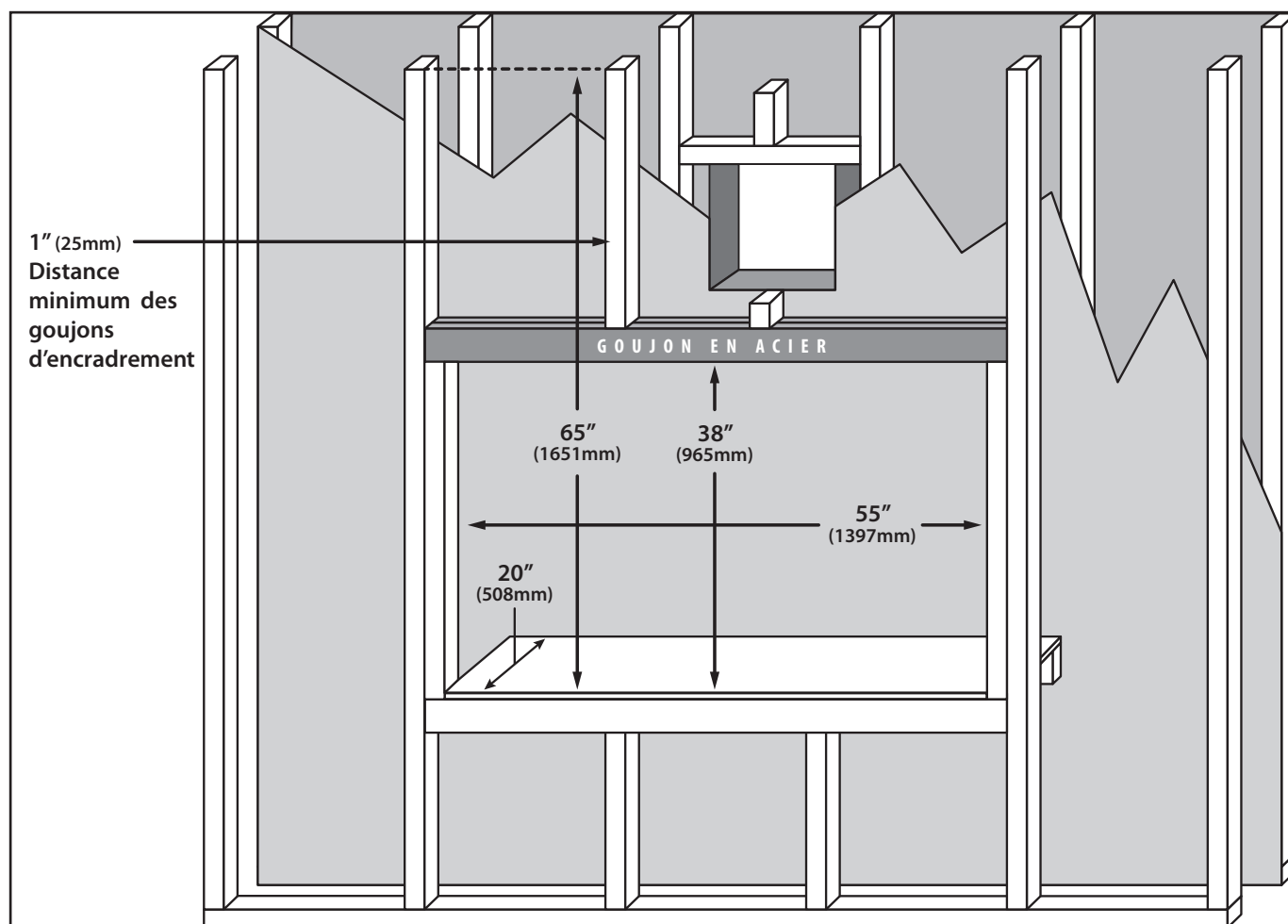
Figure 31: Dimensions de montage de charpente
