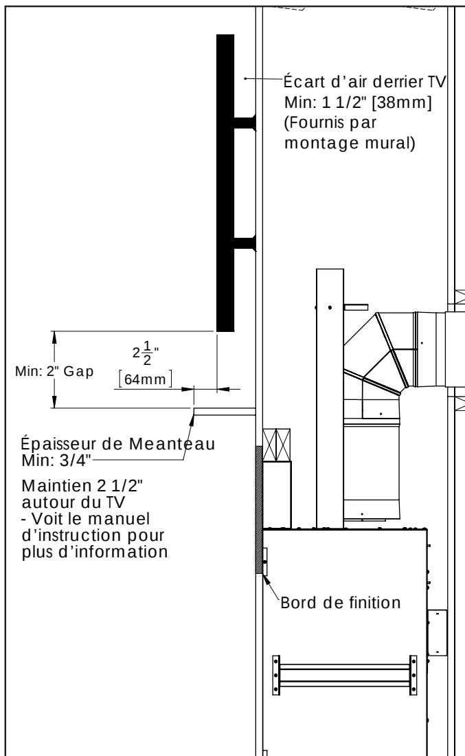
Figure 44: Dégagement Minimum d'Installation de TV
